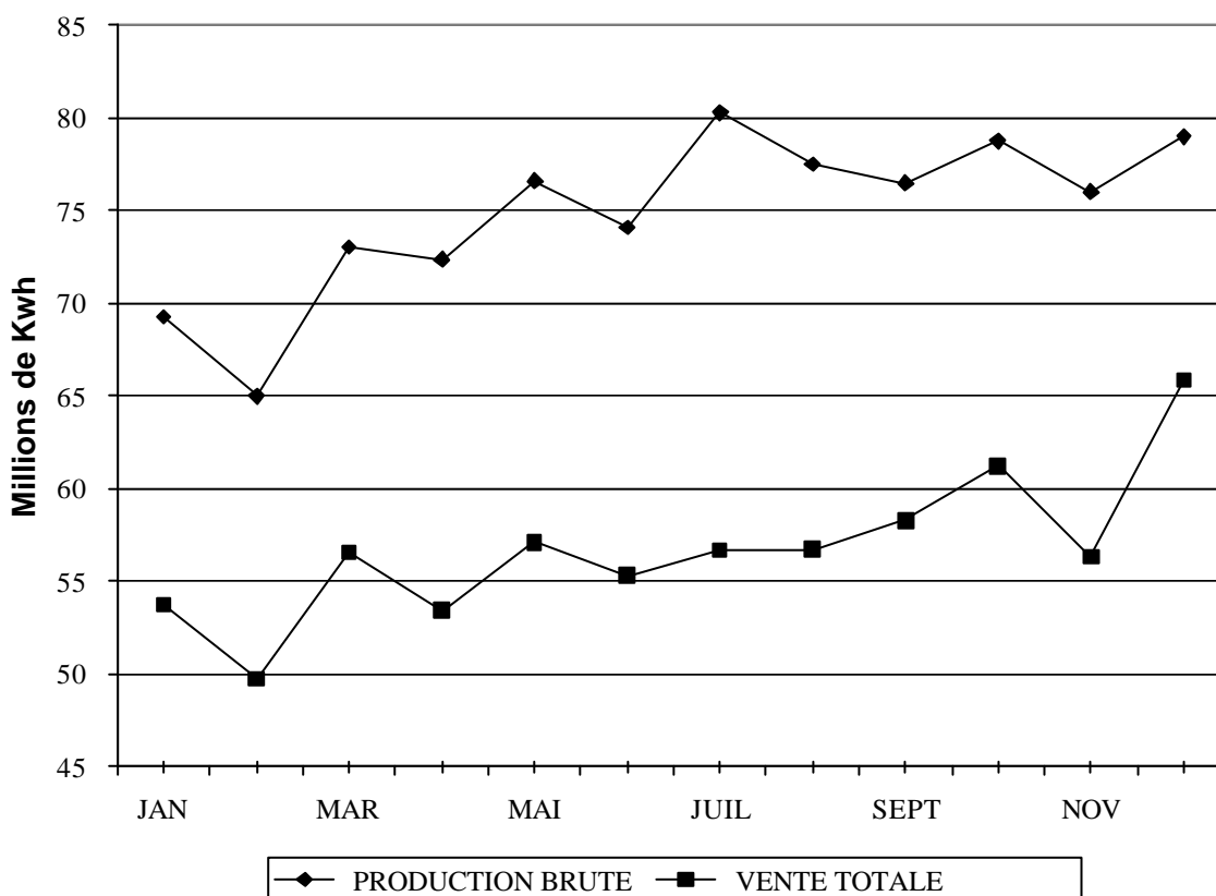
Graphique 13 : Evolution de la production et de la vente d'électricité en 2003
